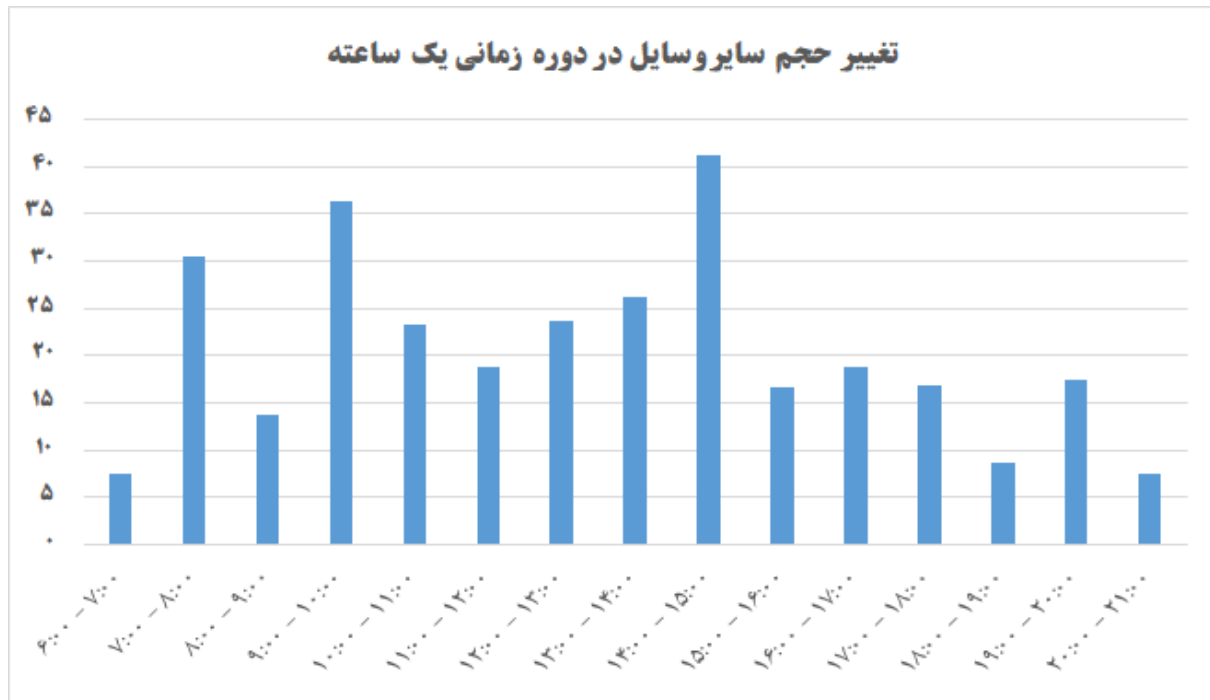
شکل ۳-۵۰: تغییرات ساعته حجم وسایل نقلیه سایر در مجموع ایستگاه های دروازه ای
