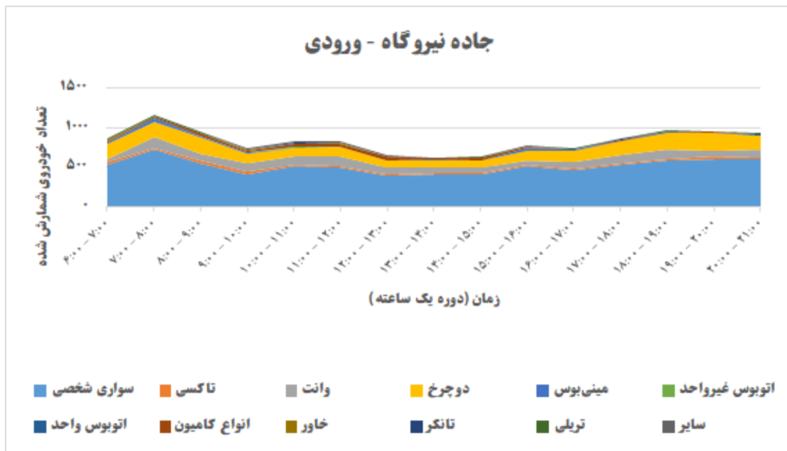
شکل ۳-۱۲: تغییرات ساحتی وسایل نقلیه ورودی از دروازه جاده نیروگاه
