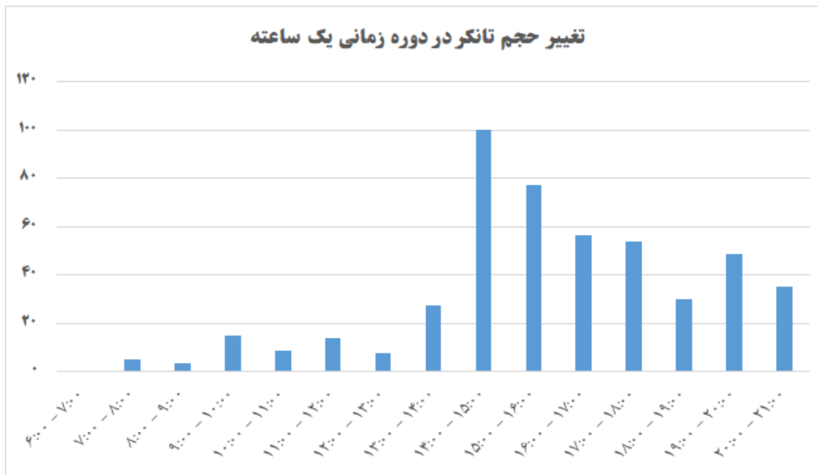
شکل ۳-۴۶: تغییرات ساعتی حجم تانکر در مجموع ایستگاه های دروازه ای
