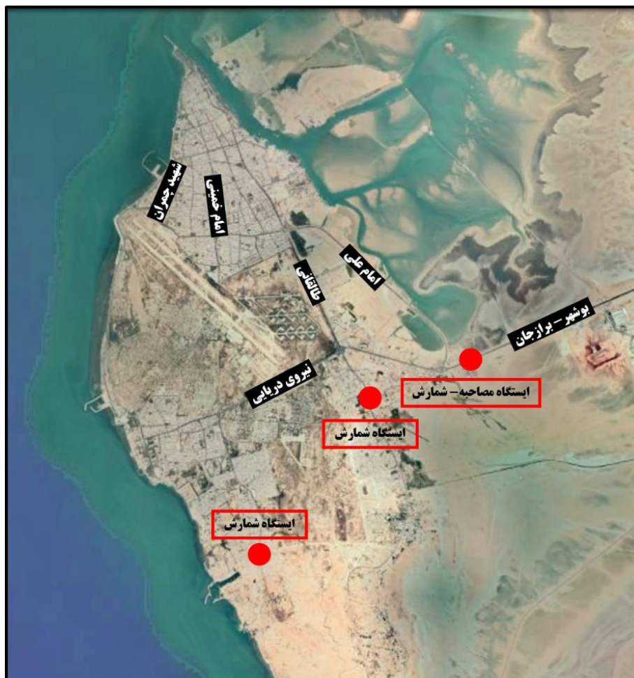
شکل ۱-۳: موقعیت ایستگاه ها در آماربرداری دروازه های شهر بوشهر
