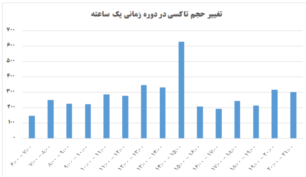
شکل ۳-۳۰: تغییرات ساعتی حجم تاکسی در مجموع ایستگاه های دروازه ای
