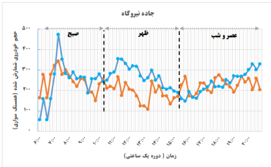
شکل ۳-۹: تغییرات زمانی کل وسایل نقلیه (همسنگ سواری) به تفکیک هر جهت در دروازه جاده نیروگاه
