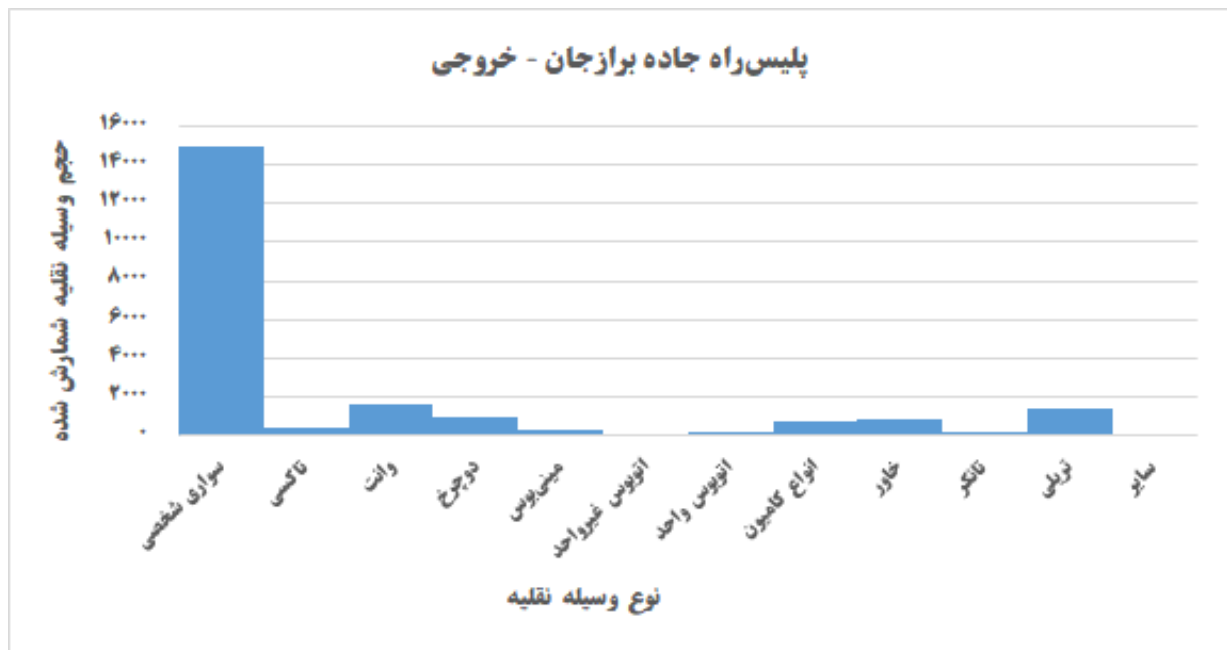
شکل ۳-۸: تعداد وسایل نقلیه شمارش خروجی از دروازه پلیس راه
