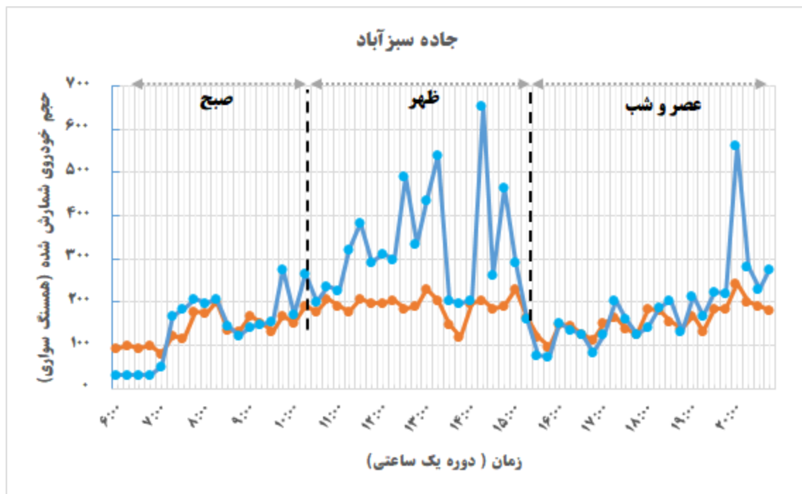
شکل ۳-۱۶: تغییرات زمانی کل وسایل نقلیه (همسنگ سواری) به تفکیک هر جهت در دروازه سبزآباد
