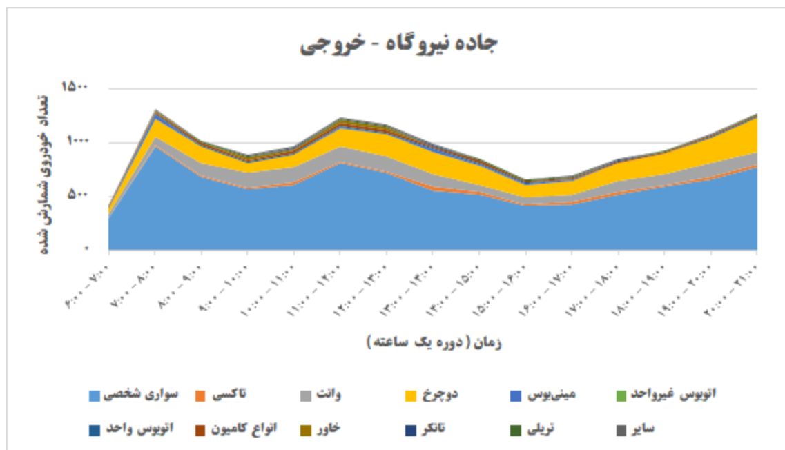
شکل ۳-۱۳: تغییرات ساحتی وسایل نقلیه خروجی از دروازه جاده نیروگاه
