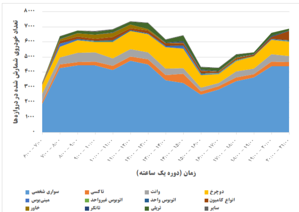
شکل ۳-۲۵: تغییرات ساختی وسایل نقلیه شمارش شده در ایستگاه های دروازه ای
