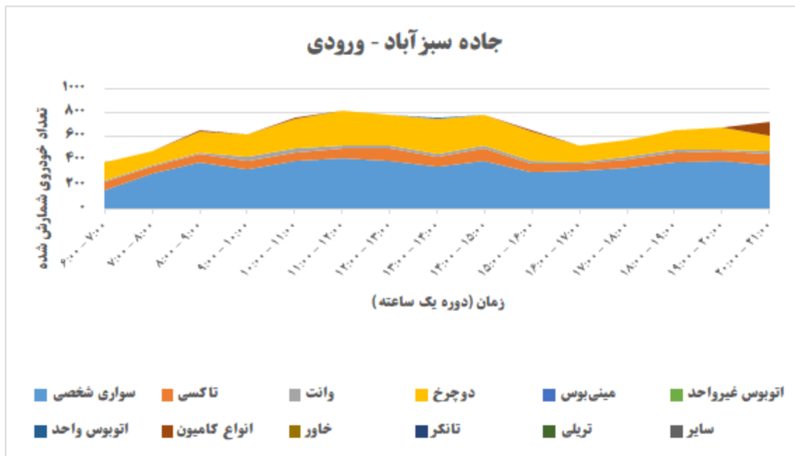
شکل ۳-۱۹: تغییرات ساعته وسایل نقلیه ورودی از دروازه سبزآباد
