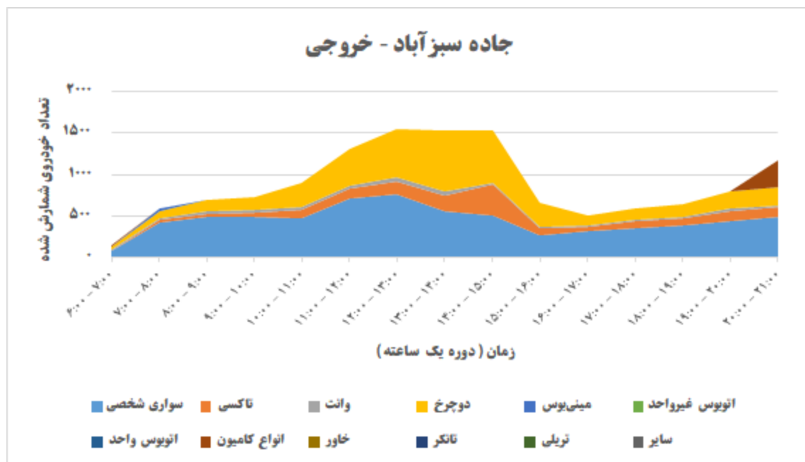
شکل ۳-۲۰: تغییرات ساعته وسایل نقلیه خروجی از دروازه سبزآباد
