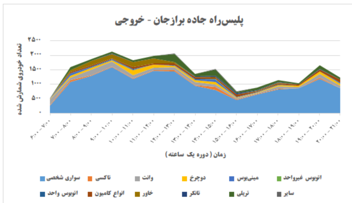
شکل ۳-۷: تغییرات ساعتی وسایل نقلیه خروجی از دروازه پلیس راه
